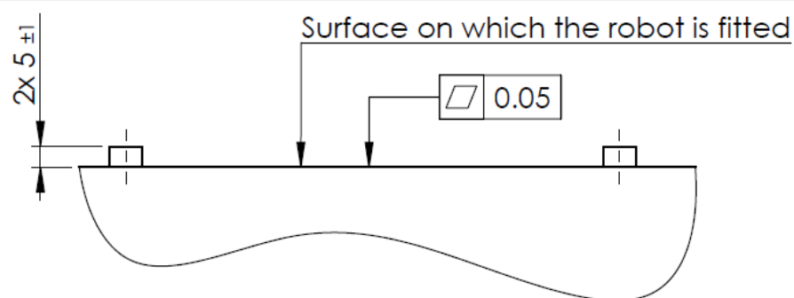
1.2: Szerelőlemez robotalaphoz
