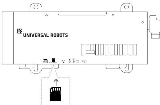
OEM vezérlődoboz
